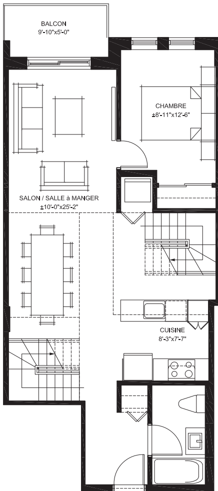
6è ÉTAGE
