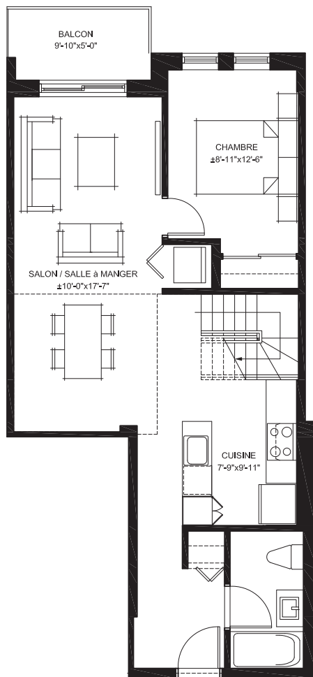
6è ÉTAGE
